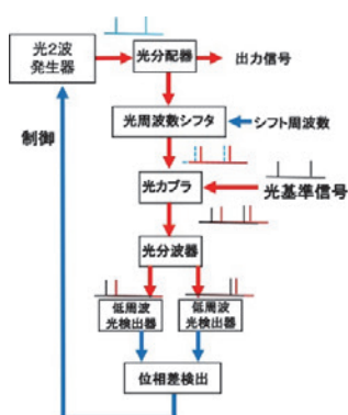
第1図 光位相同期発振器
