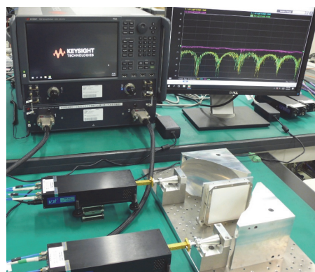
図1 自由空間法の測定系の写真
