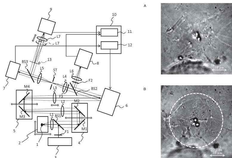
特許[4]より、左図(明細書 図.1)は、系の構成例である。右図:(明細書 図.40に加筆)は、タマネギの生細胞の核近傍の顕微鏡像である。上図(A)は通常の像で下図(B)は補償光学による補正像である。実用的な視野径(破線)で細部が \mu\text{m} 以下まで明瞭化できている。
