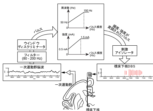
図2 今回開発した適応型DBSの装置構成
