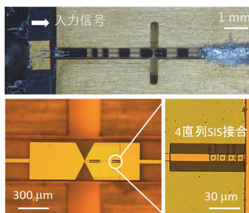
図2 実験に用いたSISミキサの写真。このSISミキサを2つ用意し、ミリ波帯の導波管を介してモジュールを従属接続することで増幅器を構成する。
