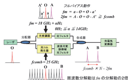
第1図 ブロック図
