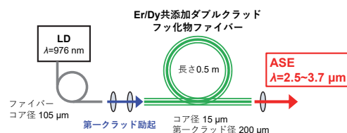
図1 開発した中赤外ASE光源の概略図
