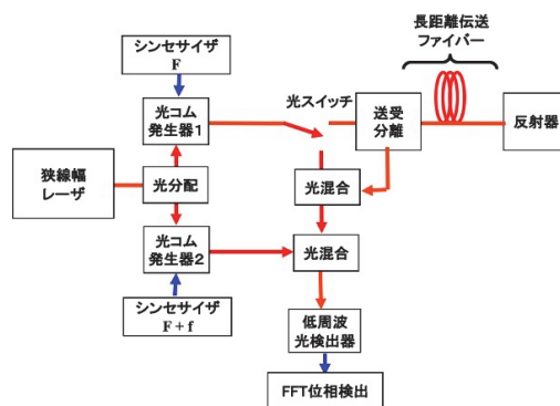
第1図 ブロック図
