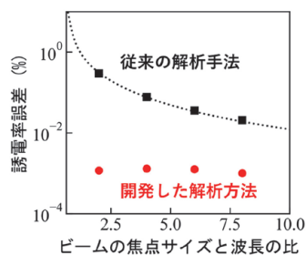
図3 電磁界シミュレーションによる解析方法の妥当性検証
