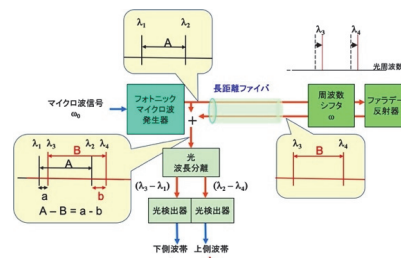
第1図 Round-trip 高周波用伝送路補償
