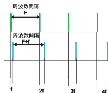
第2図 信号の周波数関係
