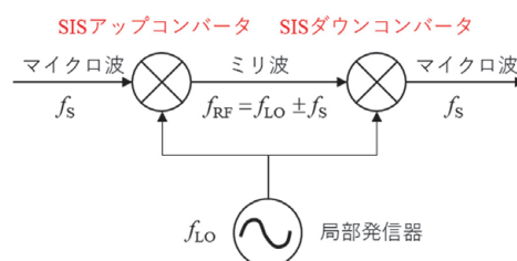
図1 考案した超伝導増幅器構成
