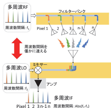
図1 多周波信号を空間マッピングするテラヘルツ波ヘテロダインイメージング装置概念図
