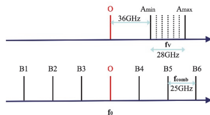
第2図 光信号の周波数関係
