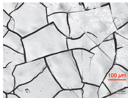
図2 急冷後の樹脂表面の顕微鏡写真
