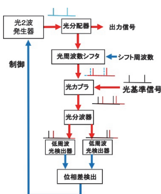
第1図 光位相同期発振器
