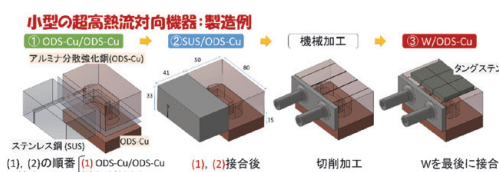
図2 先進多段階ろう付接合方法 (AMSB) による小型の超高熱流対向機器の製造例
