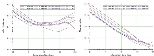
第3図 Round-trip 伝送路補償前(左) 後(右)
