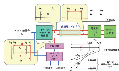
第2図 Round-trip 低周波用伝送路補償
