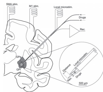
図1 サルの実験セットアップ。記録と刺激ができる電極（丸内）を、大脳基底核の淡蒼球外節（GPe）、内節（GPi）に刺入する。
