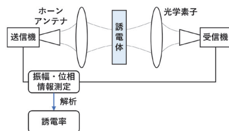
図2 自由空間法の測定系の構成
