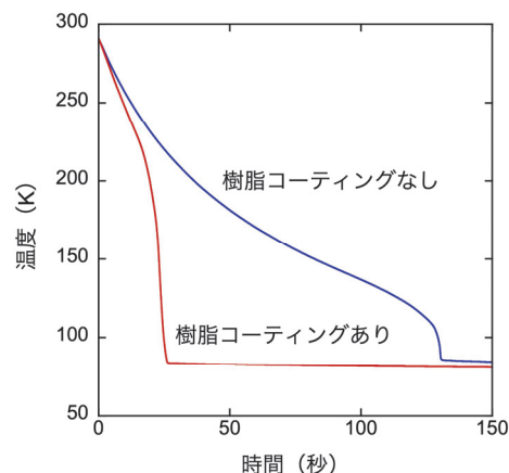
図1 樹脂コーティングした銅板の急冷実験
